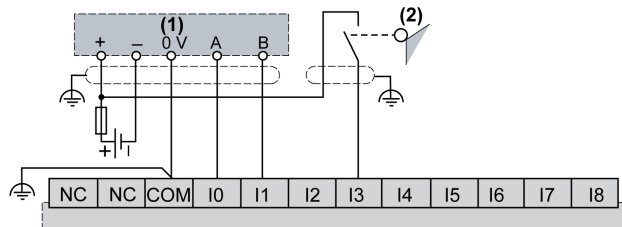
(1) Codificador de fase dual sin índice
