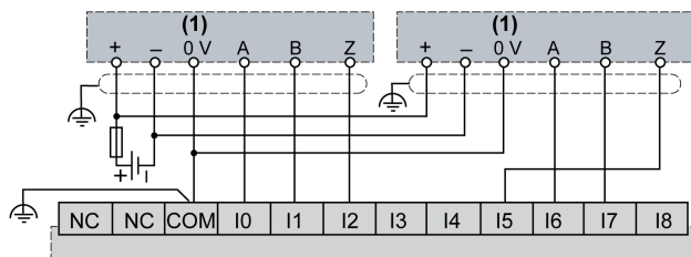
(1) Codificador de fase dual con índice
