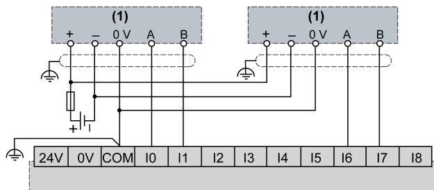
(1) Codificador de fase dual sin índice
