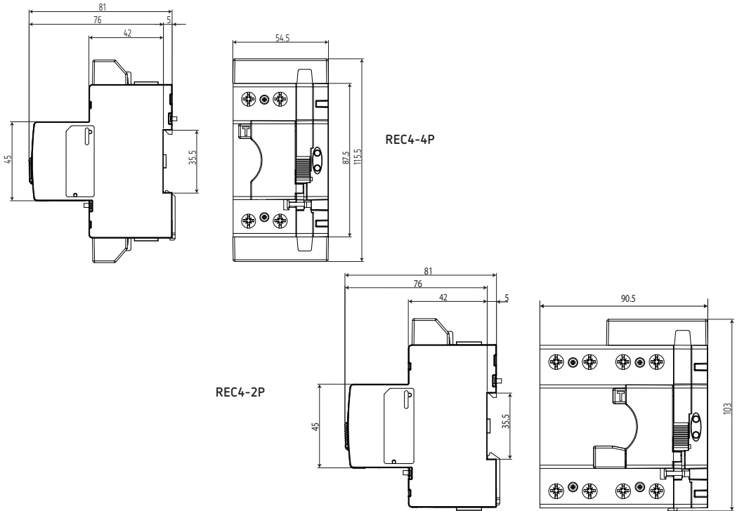
Dimensiones / Dimensions
