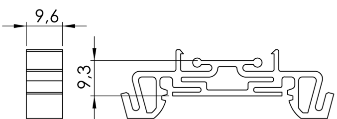
Accesorio / Accessory PA-TC/WG (mm)
