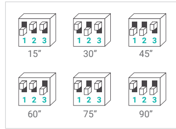
Durchflussdetektor-Modus (Sperrzeit)
