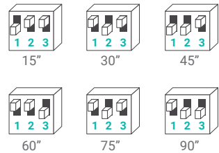
Fonction fluxostat (temps d'amorçage)
