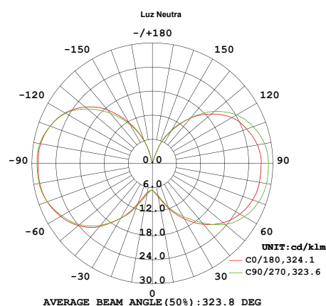
Curva de Distribución Luminosa
