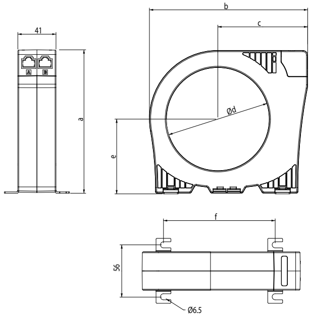
Dimensiones / Dimensions / Dimensiones / Dimension / Dimensioni / Wymiary
