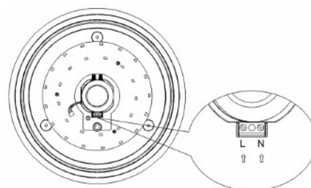
Esquema de conexión
