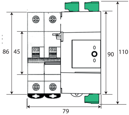
Instalación monofásica - 2 polos / Single-phase installation - 2 poles
