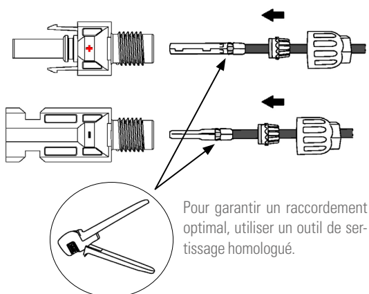
Fig. 24. Sertissage du câble.
