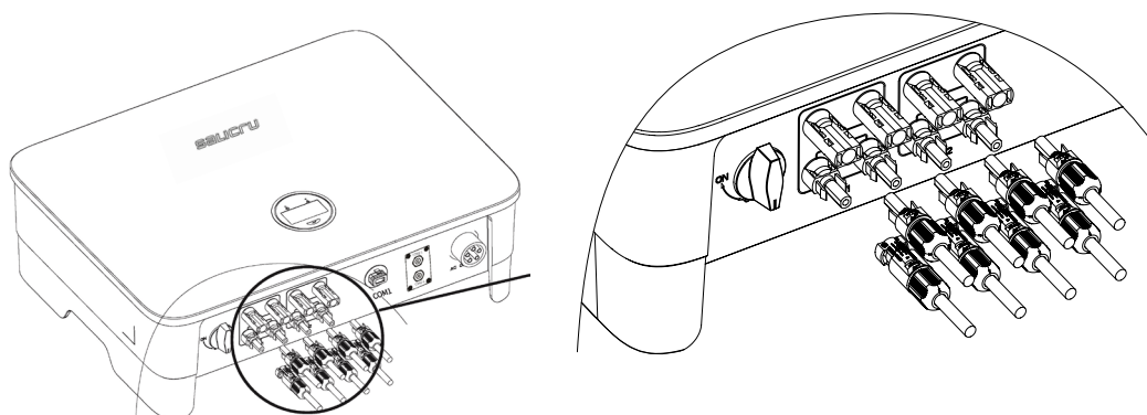
Fig. 30. Conexión terminales entrada DC equipos con 2 MPPT.
