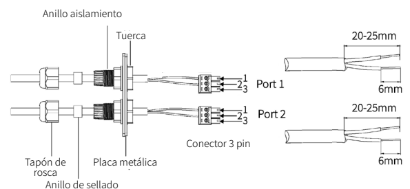
Fig. 41. Proceso de conexión al terminal.
