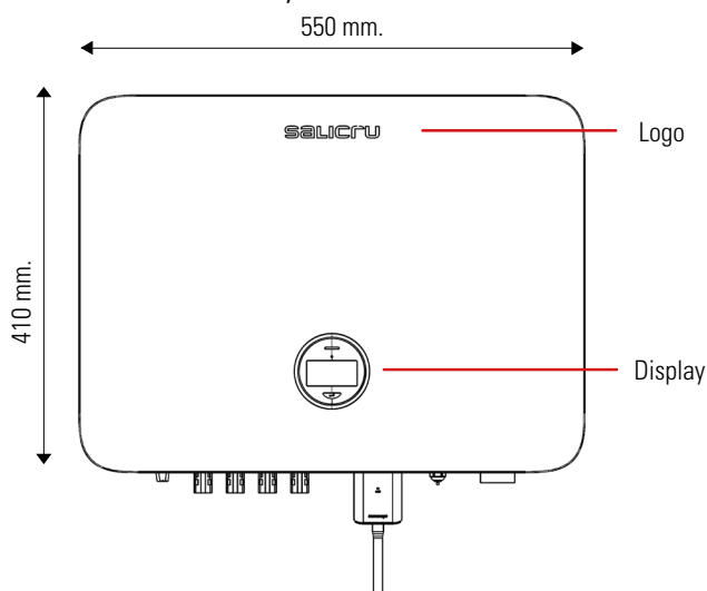
Fig. 2. Vue de face.
