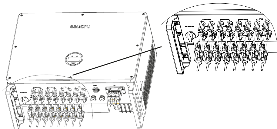
Fig. 31. Raccordement des bornes d'entrée CC sur les dispositifs à 4 MPPT
