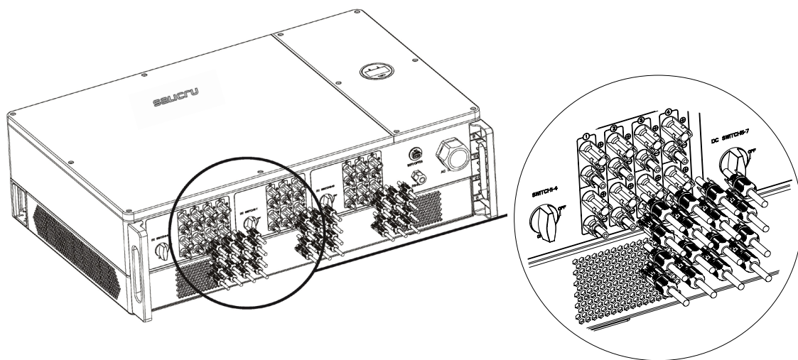
Fig. 32. Equipos con 10 MPPT.
