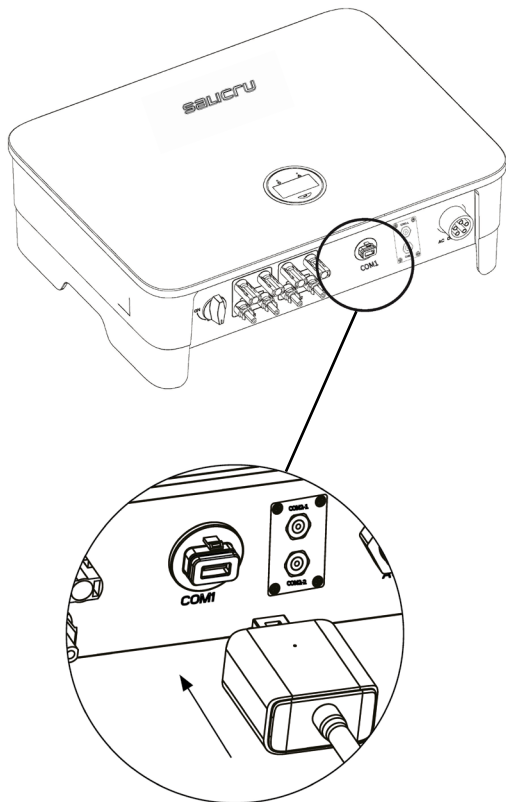
Fig. 39. Conexión dispositivo de comunicación (antena WiFi).
