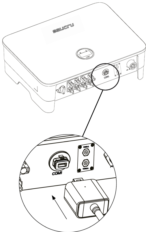
Fig. 39. Raccordement du dispositif de communication (antenne Wi-Fi).
