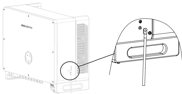
Fig. 20. Conexión del terminal de tierra.
