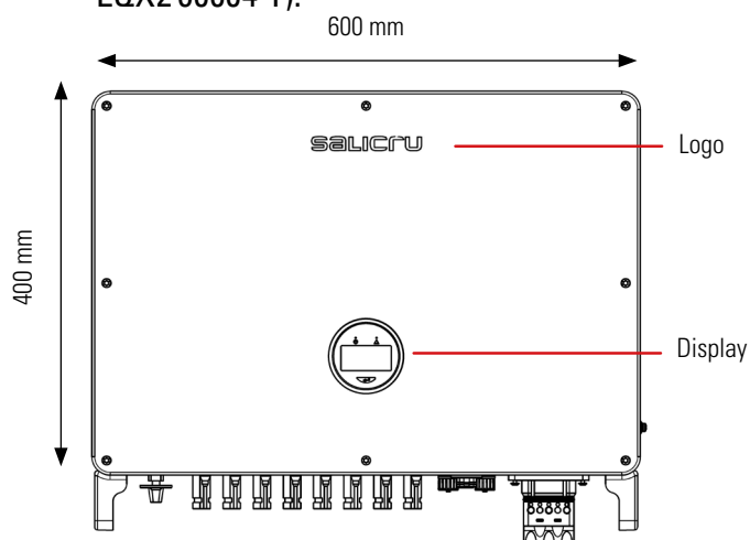
Fig. 6. Vue de face.
