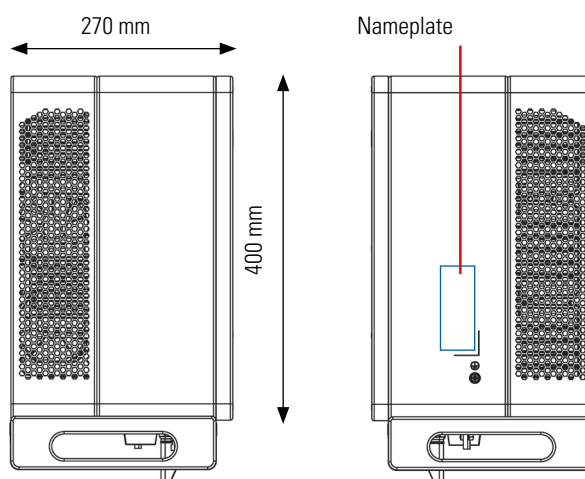
Fig. 7. Side view.
