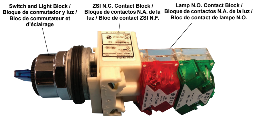
FIG. 2 : MMS Switch Assembly / Montaje del conmutador de MMS / Assemblage du commutateur MMS
