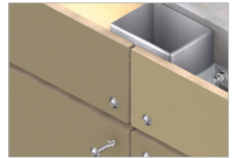
Fibro-cemento sobre acero
