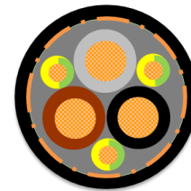
Sección del cable.
