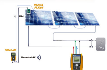
Medida de una curva I-V con sincronización a distancia de irradiación y temperatura
