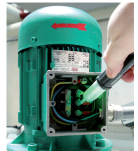
Reconocimiento de fase L2 e indicación del correcto sentido cíclico de las fases
