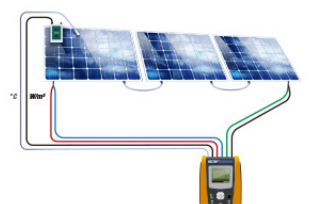
Medida de una curva I-V con sensores ambientales conectados al I-V500w
