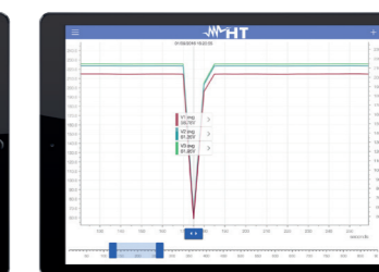
Ejemplo de visualización Registro efectuado (Evidentes huecos de tensión)
