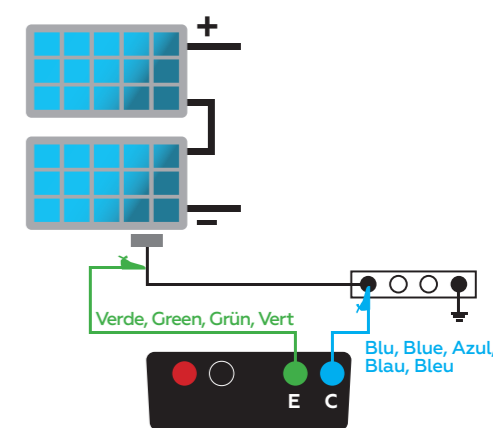
FUNCIÓN RPE Esquema de conexión
