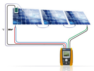
Medida de una curva I-V con sensores ambientales conectados al I-V500w
