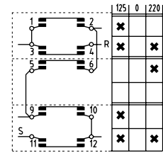
317 Arranador monofásico 2 tensiones 3 pisos
