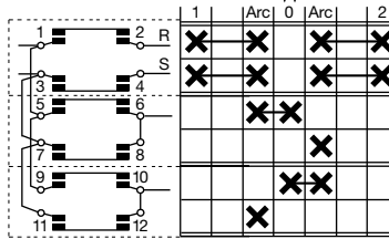
316 Arranador inversor del T315 1 - ARR - 0 - ARR - 2 3 pisos
