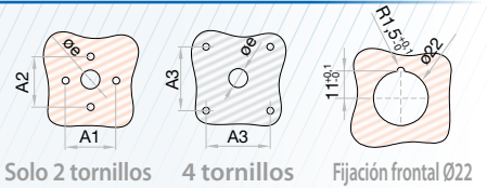
Solo 2 tornillos 4 tornillos Fijación frontal Ø22
