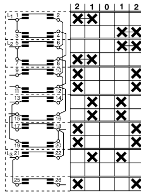
332 Dahlander inversor del T330 7 pisos
