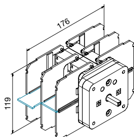
Separadores horizontales Código DT-90026 (2 unidades)
