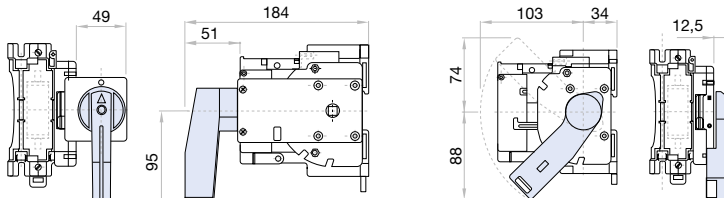
mando directo frontal
