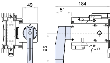
mando directo frontal
